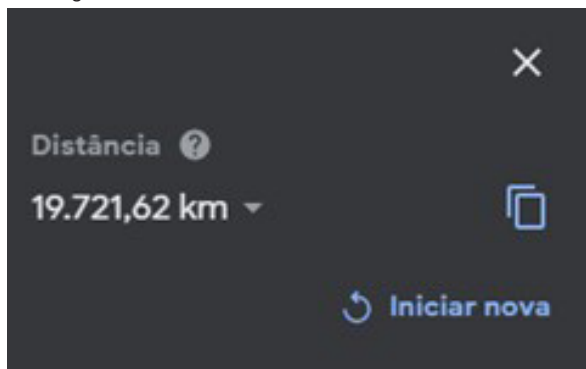
Figura 13: Verificando a distância entre Curitiba e Uruma.
