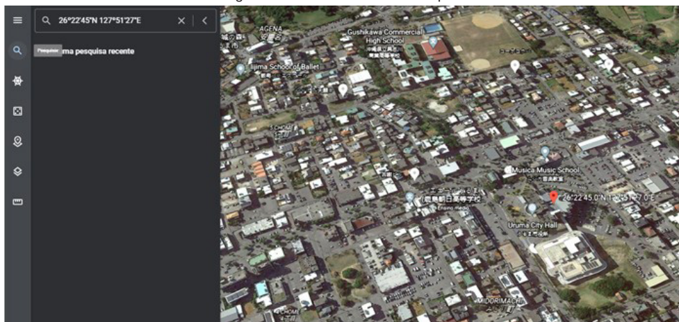
Figura 10: Localizando Uruma no Japão.
