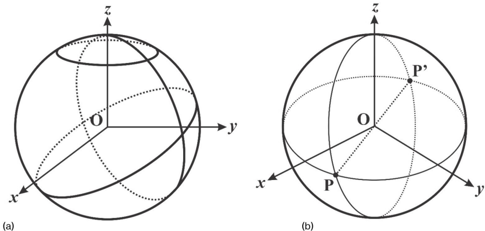
Figura 2: Circunferências de S_\rho^2 : (a) mínimas; (b) máximas.
